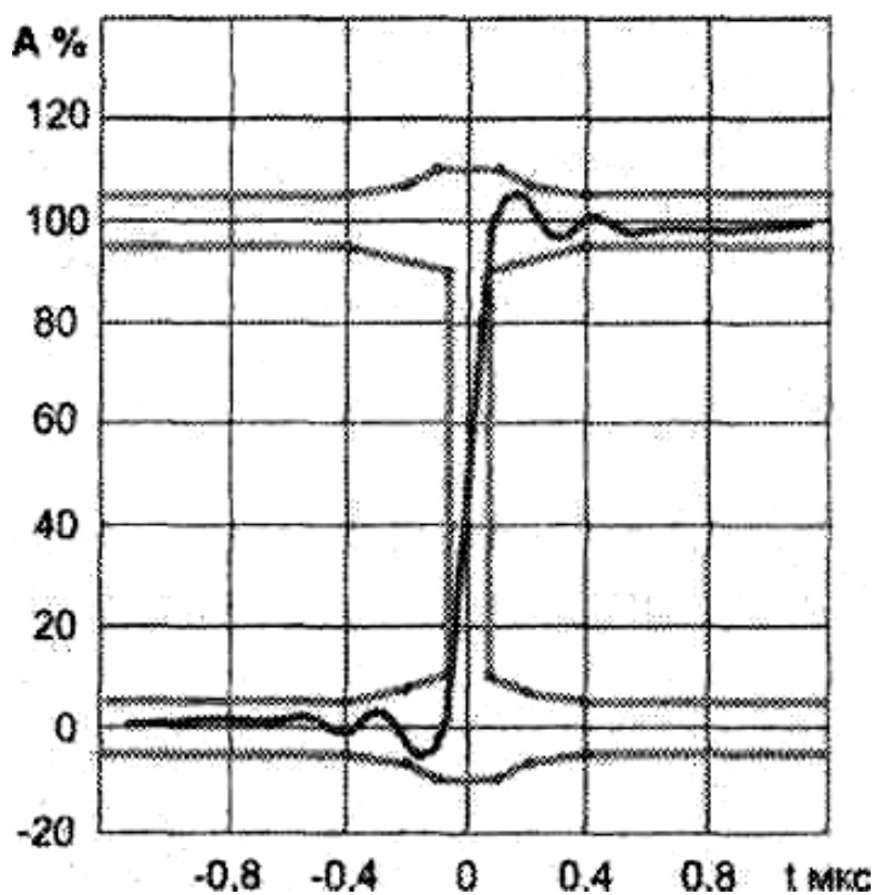
Рис. Г1 - Шаблон, внутри которого укладывается переходная характеристика.
