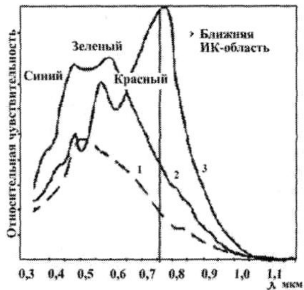
Рис. А2 - Спектральные характеристики чувствительности ПЗС:
