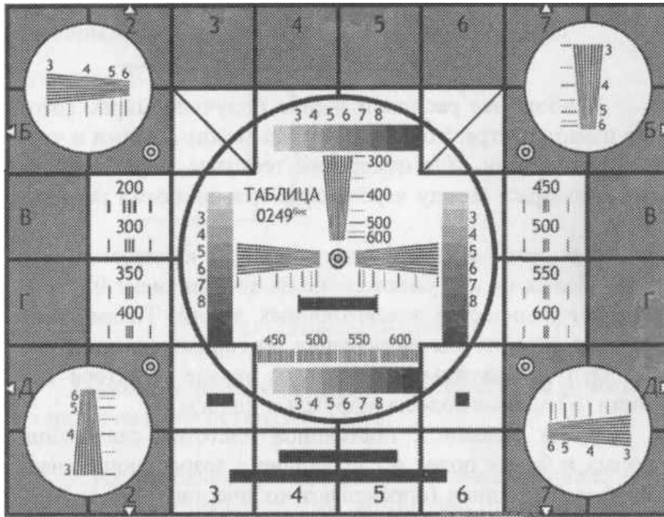
Рис. Б1 - Тестовая испытательная таблица «ТИТ-0249»
