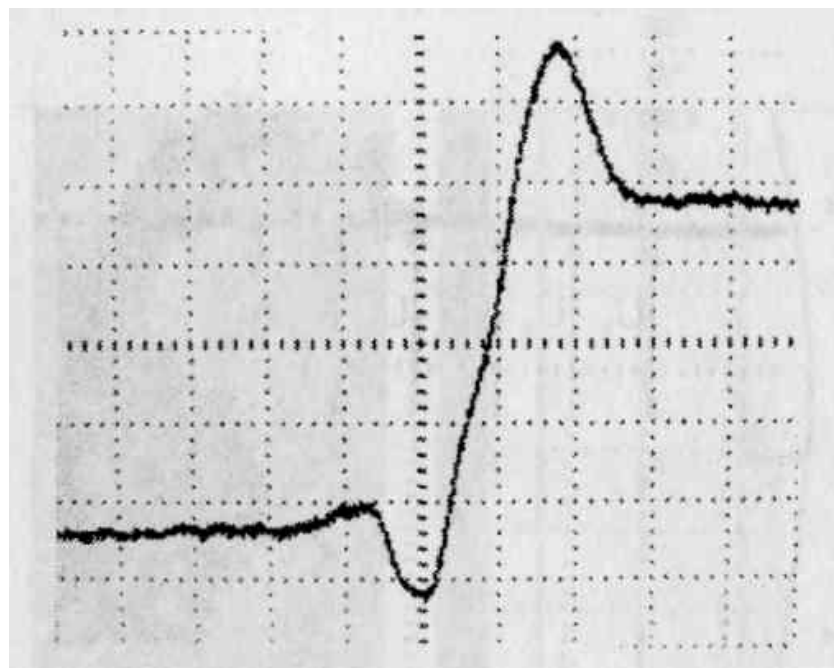
Рис. Г8 - Реальные эпюры напряжения от телекамеры в точке 4. (см. Рис. Г3) Переходная характеристика с черного фона на белый.
