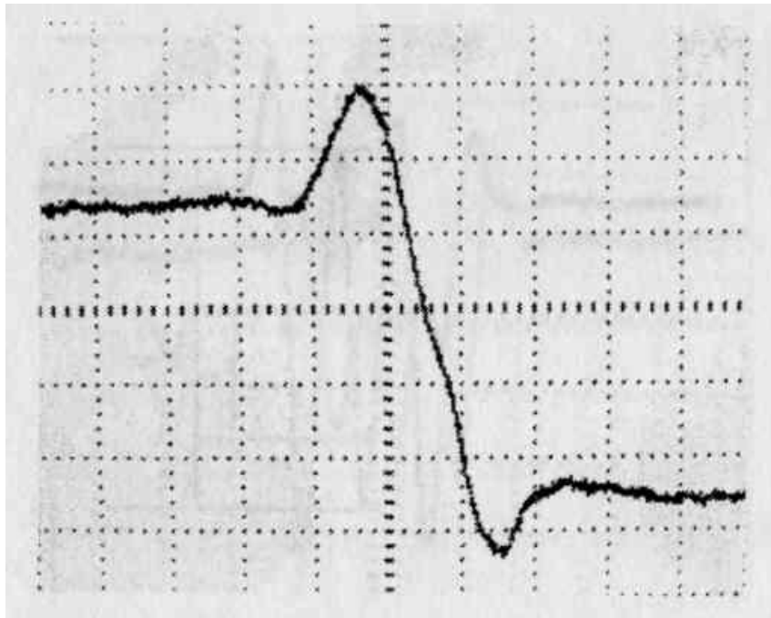
Рис. Г7- Реальные эпюры напряжения от телекамеры в точке 5. (см. Рис. Г3) Переходная характеристика с белого фона на черный.
