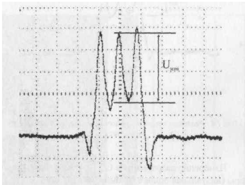
Рис. Гб - Реальные эпюры напряжения от телекамеры в точке 3 (см. Рис. Гз)
