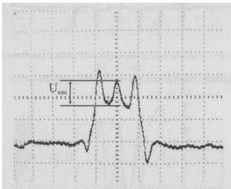
Рис. Г4 - Реальные эпюры напряжения от телекамеры в точке 1 (см. Рис. Г3)
