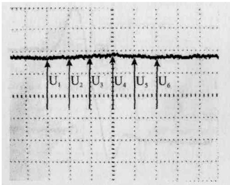
Рис. ПО- Реальные эпюры напряжения от телекамеры в точке 7
