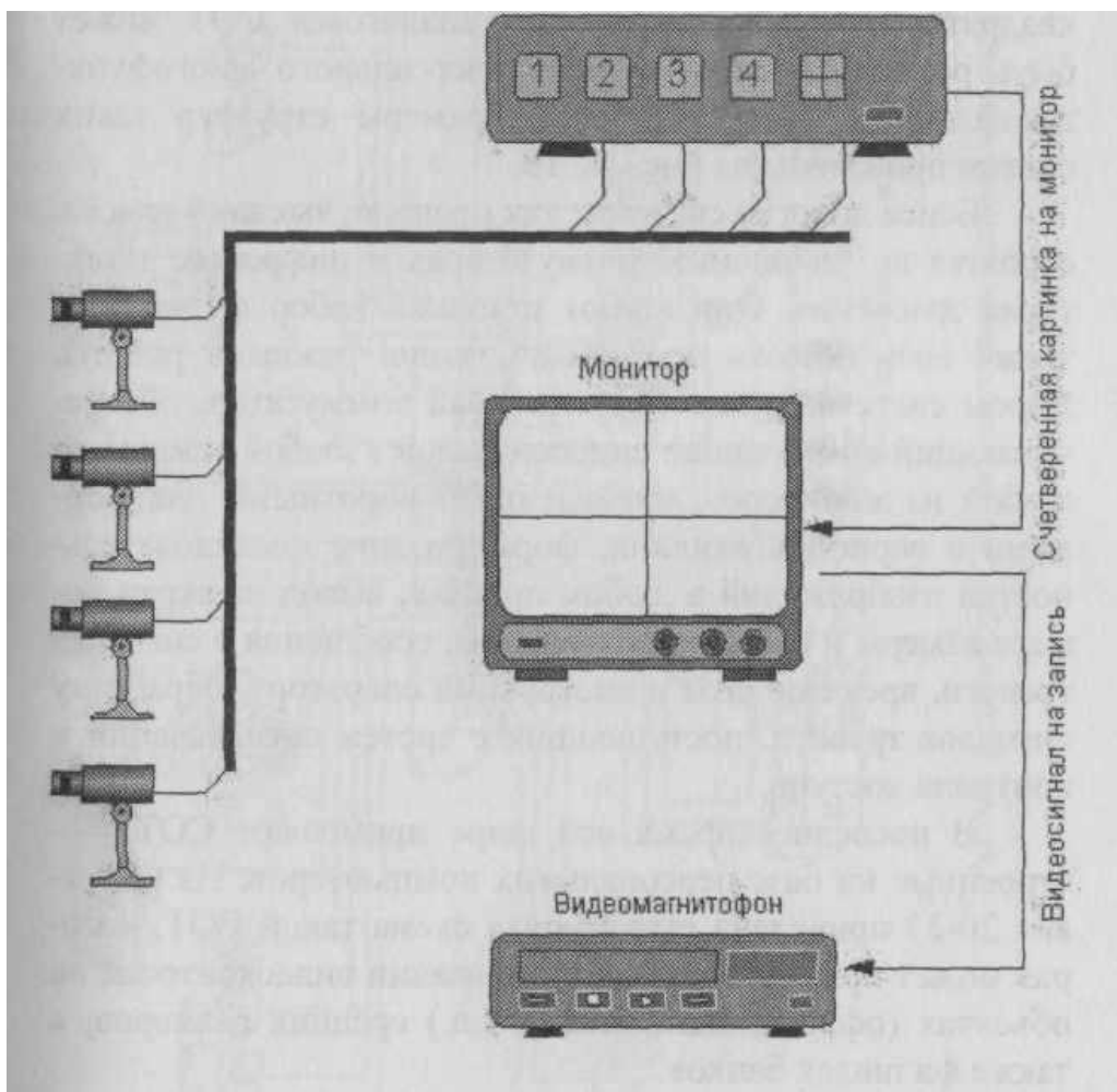
Рис. 7 - Структурная схема системы видеонаблюдения с квадратором
