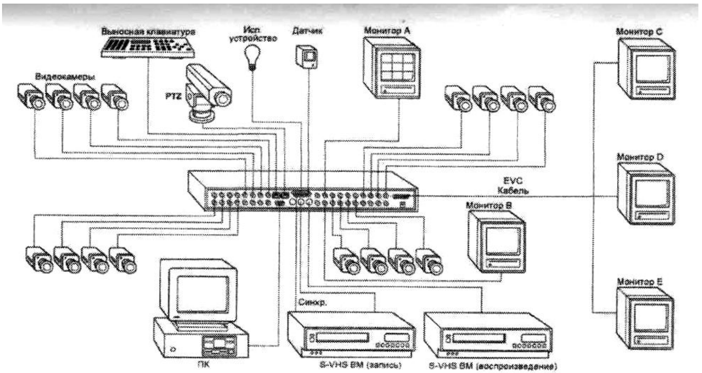
Рис.18 - Структура COT на базе универсального мультиплексора
