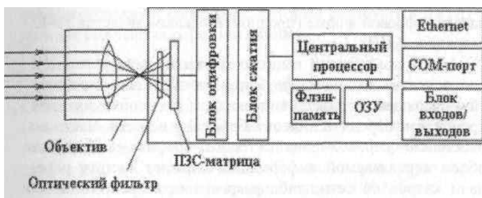
Рис. 10- Устройство IP-камеры
