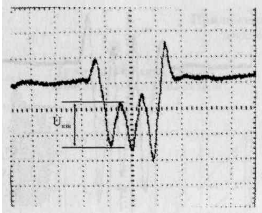
Рис. Г11 - Реальные эюры напряжения от телекамеры в точке 8 (см. Рис. Г3)
