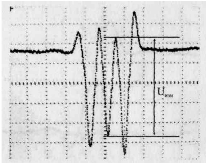
Рис. Г9 - Реальные эпюры напряжения от телекамеры в точке 6.
