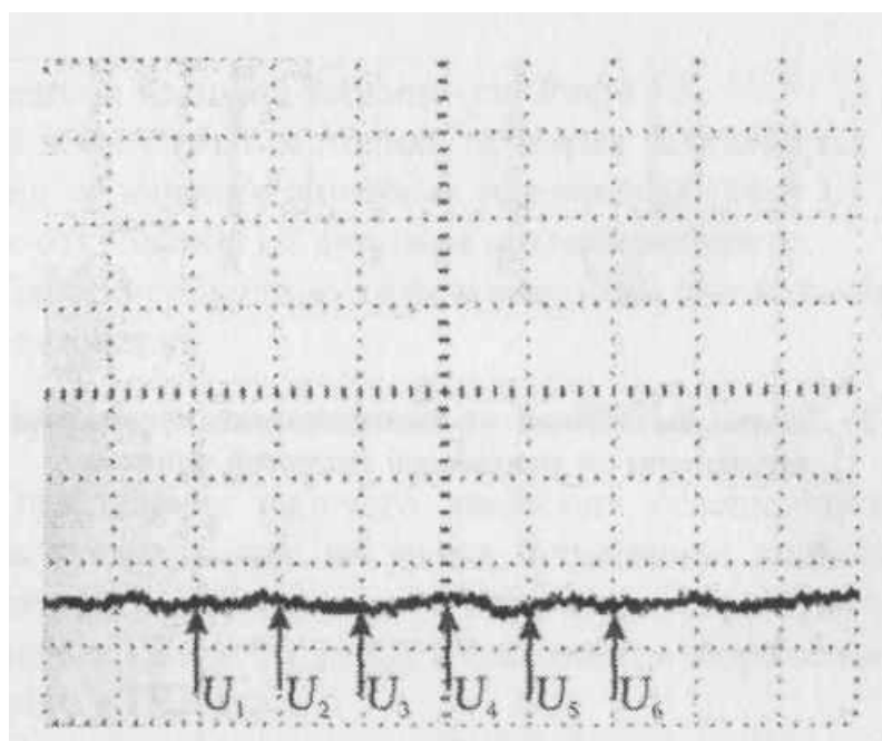
Рис. Г5 - Реальные эпюры напряжения от телекамеры в точке 2 (см. Рис. Г3)
