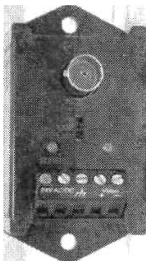
Рис. Н5 - Внешний вид активного передатчика по «витой паре» (вид сверху) В центре виден переключатель длины линии 500 м, 1000 м, 1600 м
