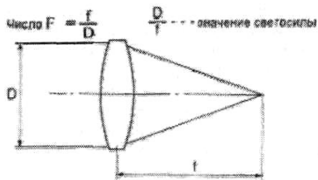
Рис. А3 - Светосила объектива
